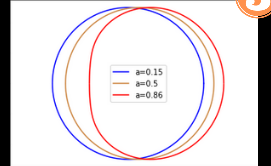
Representación gráfica de la sombra de un agujero negro de Kerr-Newman
