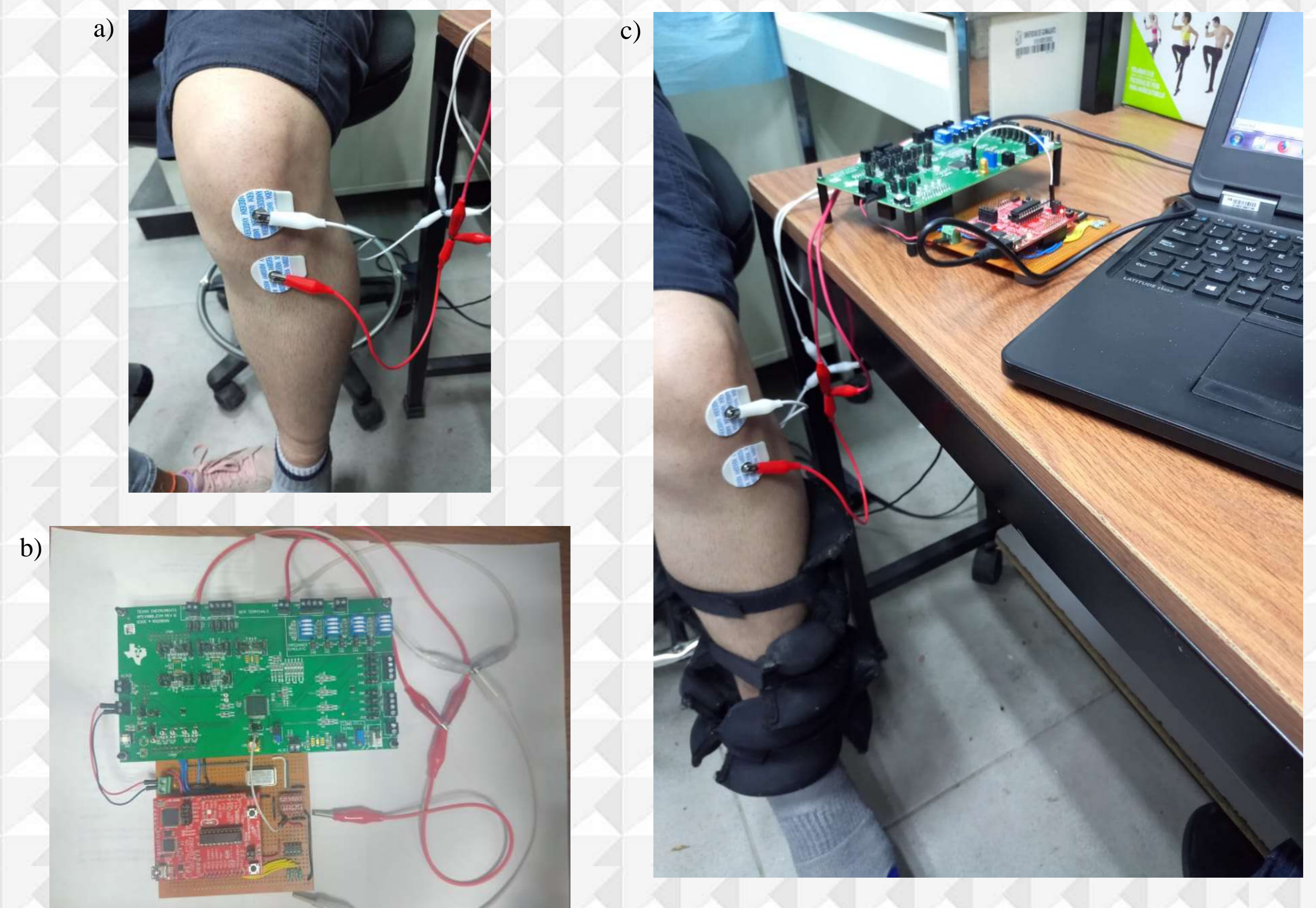
Figura 1. Montaje del sistema experimental a) Colocación de electrodos a lo largo del tendón rotuliano b) Sistema EBMS-DIF-DCI-UG c) Montaje del experimento rodilla-equipos de impedancia.
